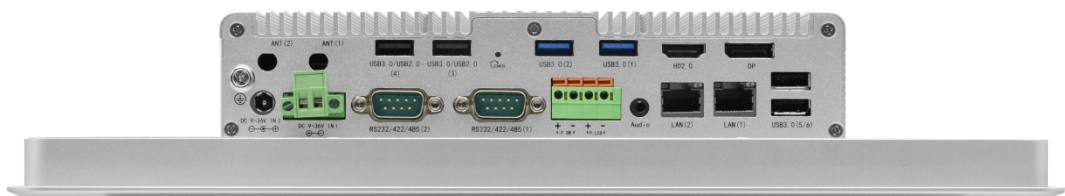
底部I/O视图
